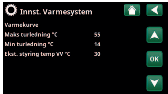
Meny «Avansert/Innstillinger/Varmesystem» ved fjernstyring til ekstern varmtvannstank.
