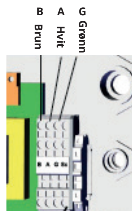
Tilkobling EcoLogic S til terminal (EcoAir)
